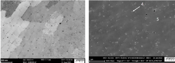
Abb. 2: REM-Untersuchung des Gefüges des aus beschichtetem CuNiSiCr hergestellten Teils. Oxiddispersion und Ausscheidungen in der Matrix sichtbar. a) CuNiSiCr-Legierung mit Cr-Beschichtung; b) Legierung mit Nb-Beschichtung, EDX Messpunkte. 5: Cu, Cr / 4: Cu, Cr, Nb
