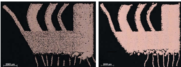
Abb. 3: Metallographische Untersuchung des aus ReinCu hergestellten Testteils (Prozessparameter 380 W, 600 mm/s, Spurabstand = 0,065 mm) Links: ReinCu, Porosität 15,9 %; rechts: ReinCu + W, Porosität 0,9 %
