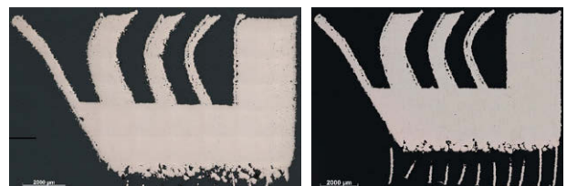
Abb.1: Metallographische Untersuchung des aus beschichtetem Cu-Legierungen hergestellten Testteils. a): CuCrZr + Nb, Prozessparameter 250W, 600 mm/s, Spurbstand = 0,055 mm, Porosität 0,02 %. b) CuNiSiCr + Cr, Prozessparameter 200W, 900 mm/s, Spurbstand = 0,055 mm, Porosität 0,04%
